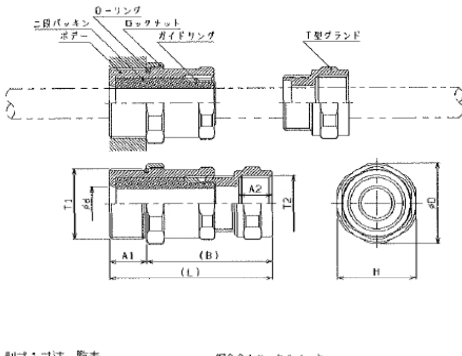
型式：寸法一覧表
